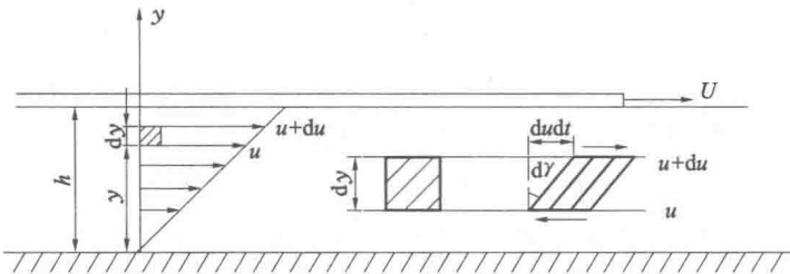
图 1.3 黏滞性实验
