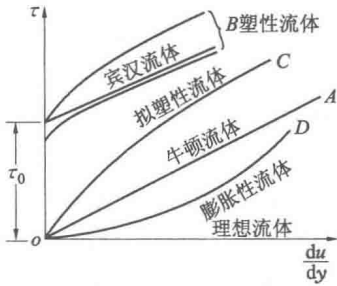
图 1.4 非牛顿流体的流动曲线
