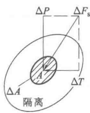
图 1.1 表面力
