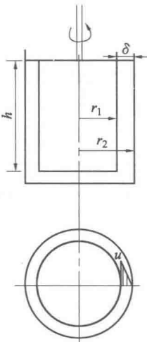
图 1.5 旋转黏度计
