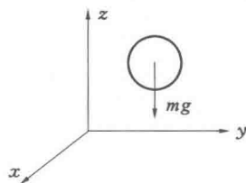
图 1.2 重力
