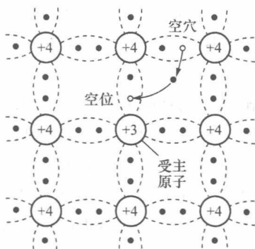
图 1.1.4 P型半导体
