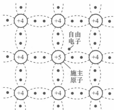
图 1.1.3 N型半导体
