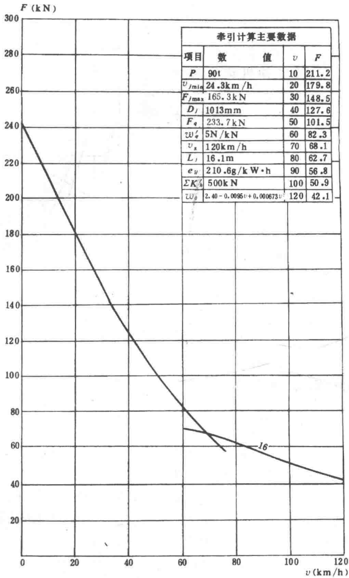
图 1-6 BJ 型液力传动内燃机车的牵引特性
