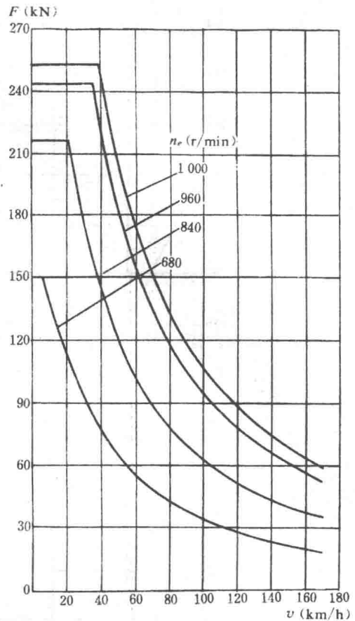
图 1-5 DF 11 型电传动内燃机车的牵引特性
