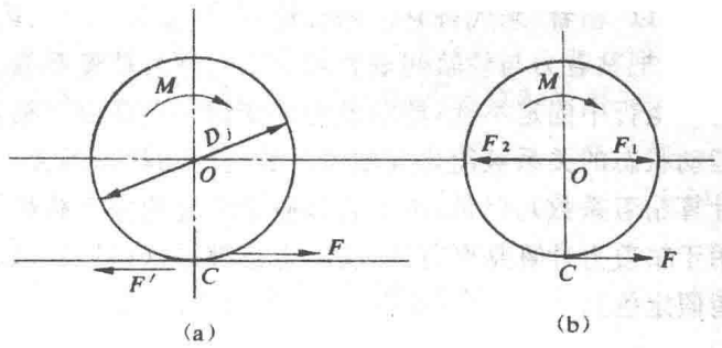
图 1-2 轮周牵引力的产生
