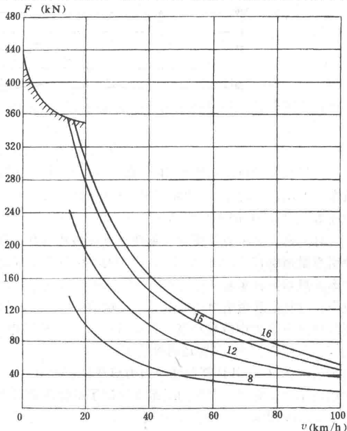
图 1-3 DF_4 (货)型电传动内燃机车的牵引特性
