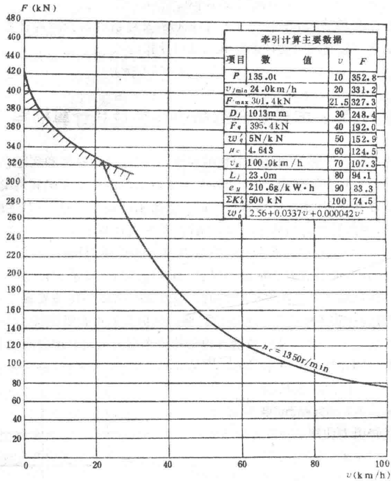
图 1-4 ND 4 型电传动内燃机车的牵引特性
