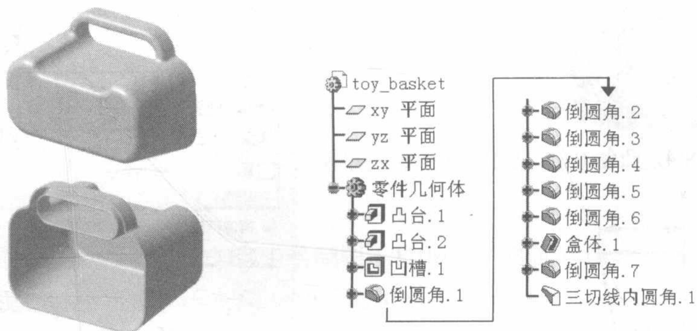
图 1.1 零件模型和特征树
