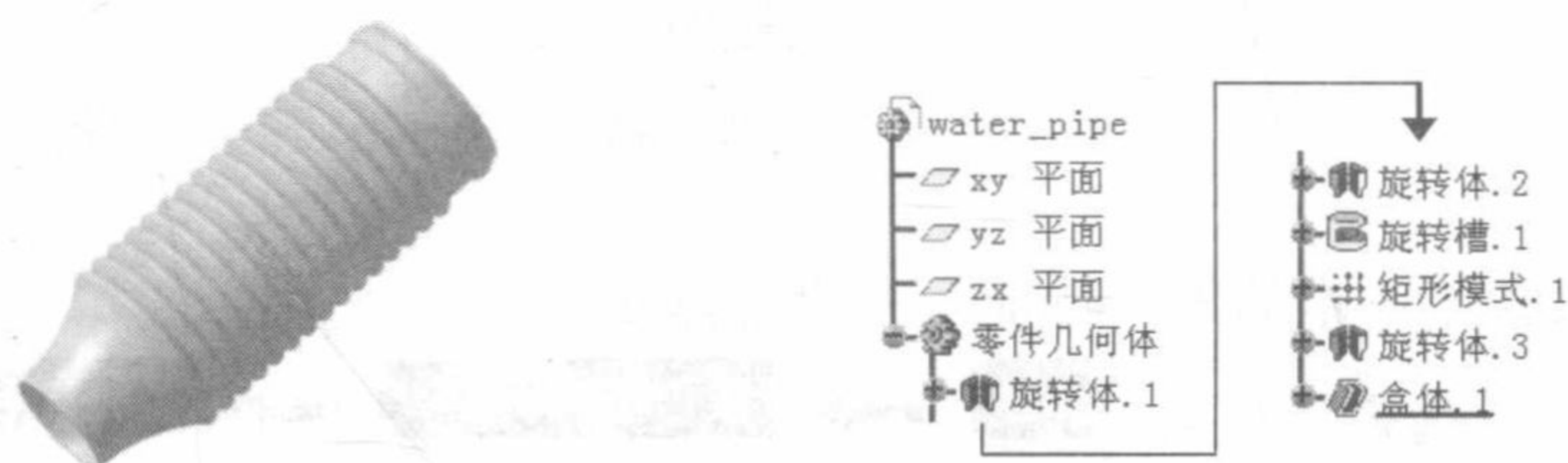
图 2.1 零件模型和特征树
