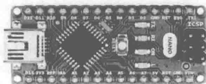
图 1-8 Arduino NANO
