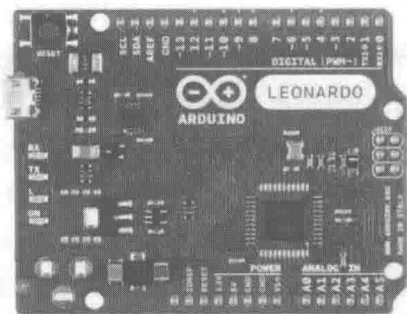
图 1-5 Arduino Leonardo
