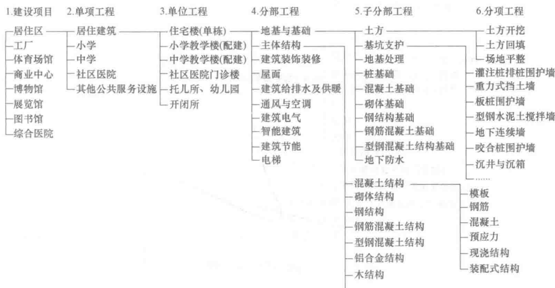
图 1-1 建设项目组成示意图
