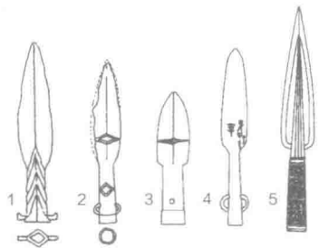
▲ 商代柳叶形铜矛。1、2为商前期款，长度约23.6厘米；3、5为中期款，分别长17.4厘米、37厘米；4为晚期款，长23.5厘米
