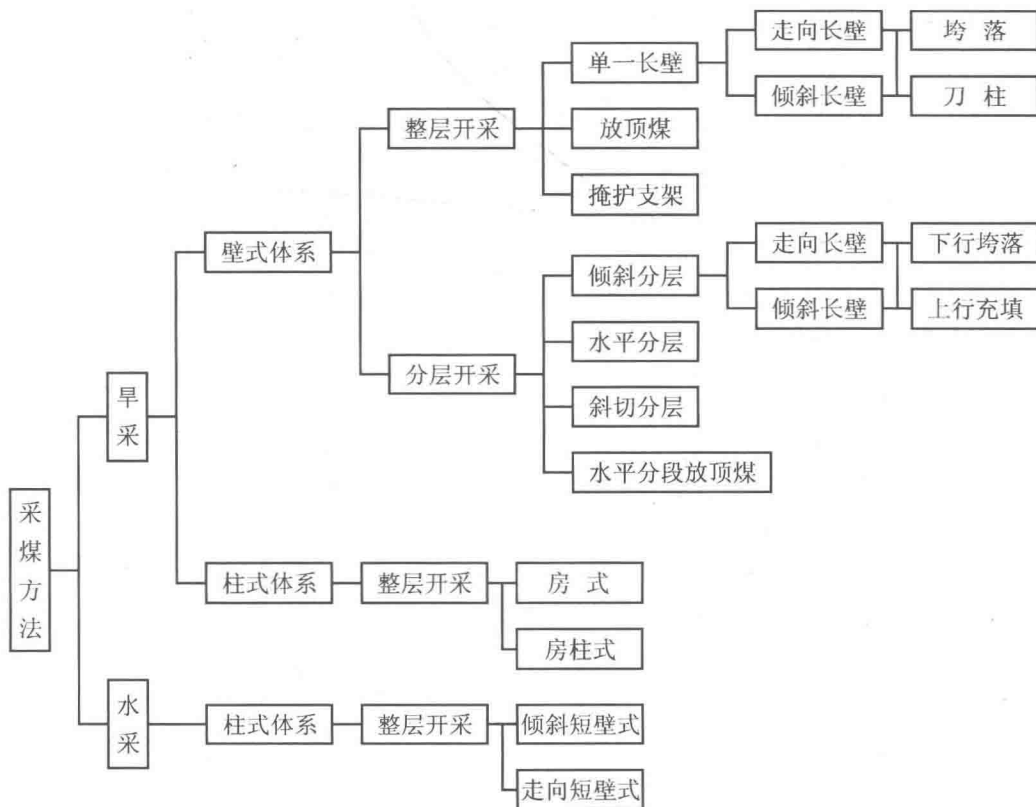
图 1-1 我国矿井开采的主要采煤方法
