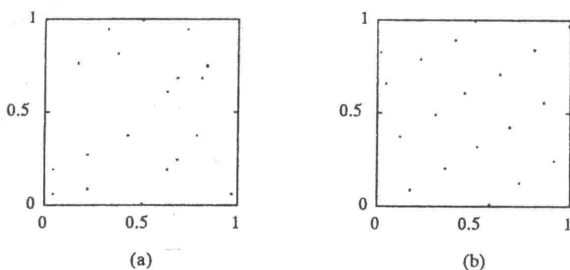
图 1.1 由蒙特卡罗方法与 NTM 生成点集的位置
