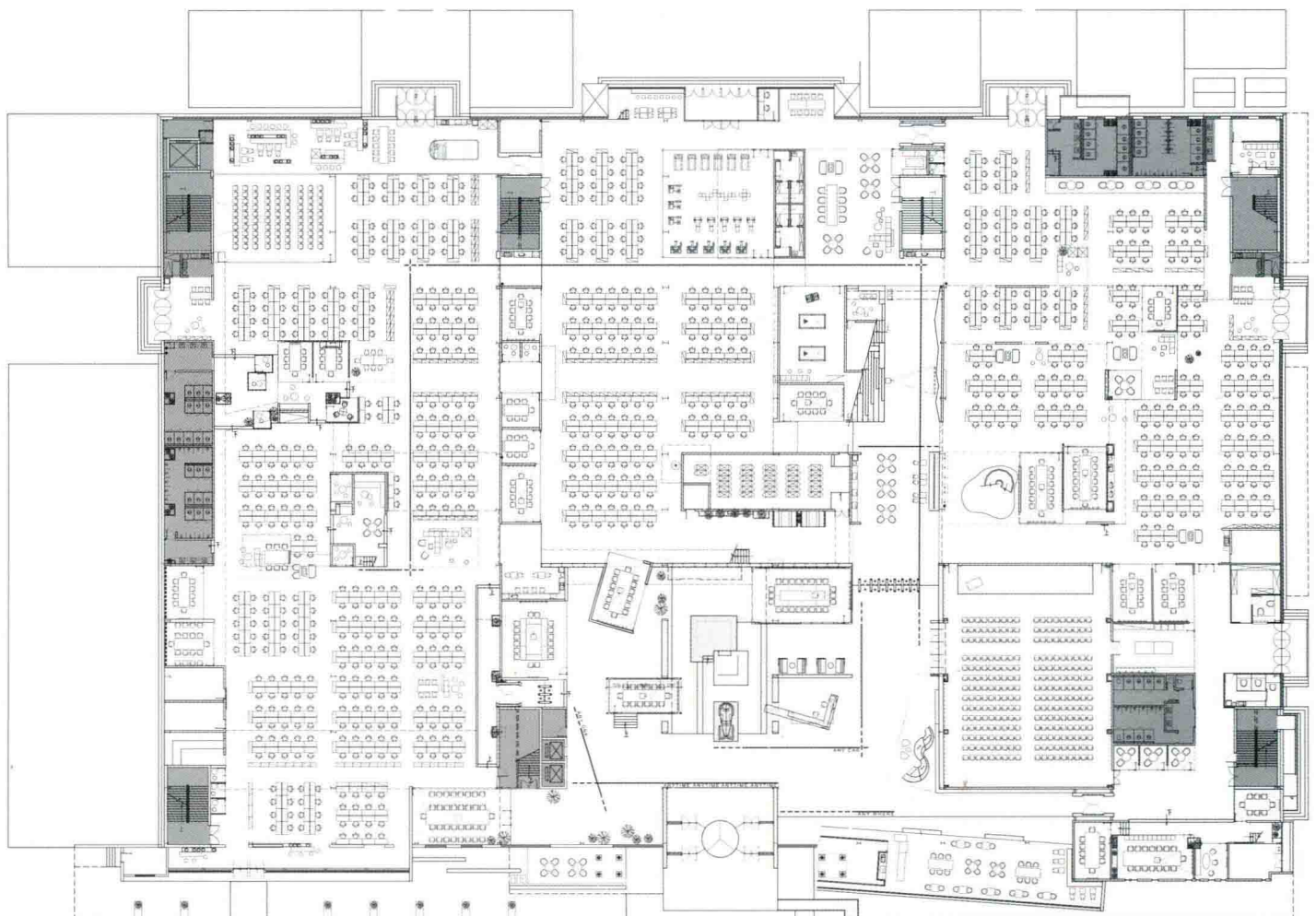
一层平面图
