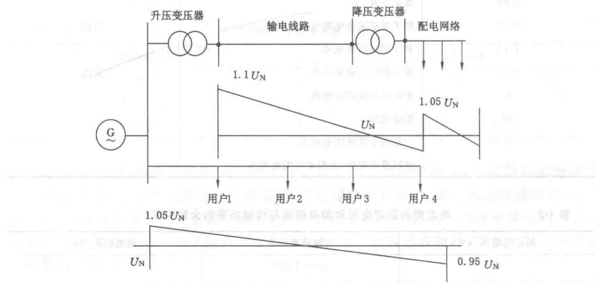
图 1-2 电力网各部分电压分布示意图
