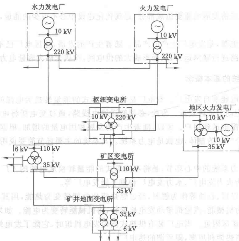
图 1-1 典型电力系统
