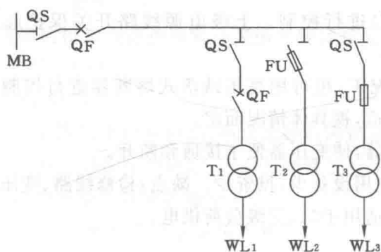
图 1-4 干线式直接连接
