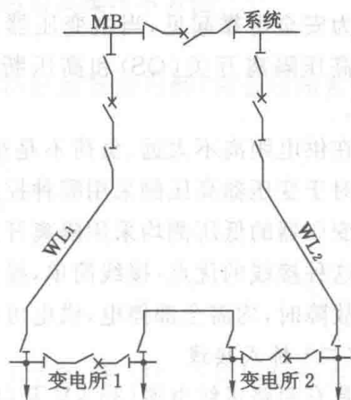
图 1-5 环式接线
