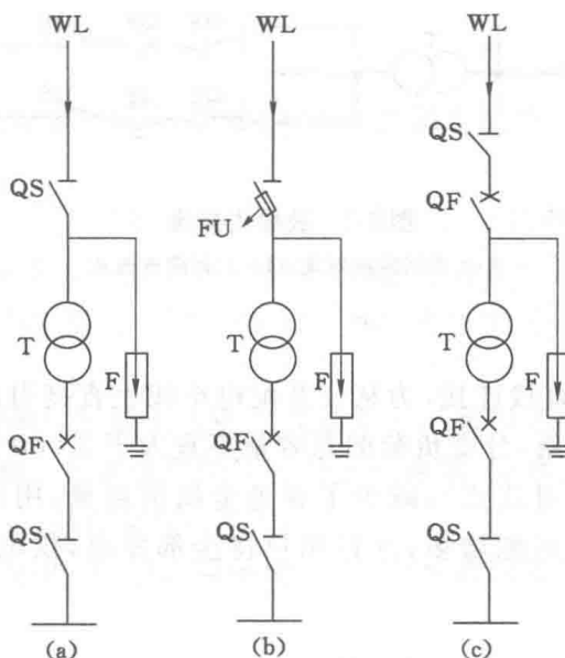
图 1-6 线路—变压器组接线
