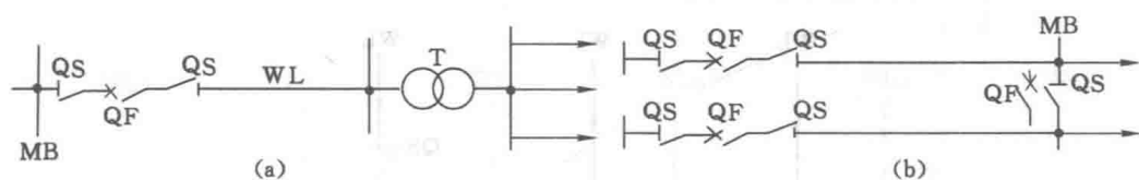
图 1-3 放射式接线
