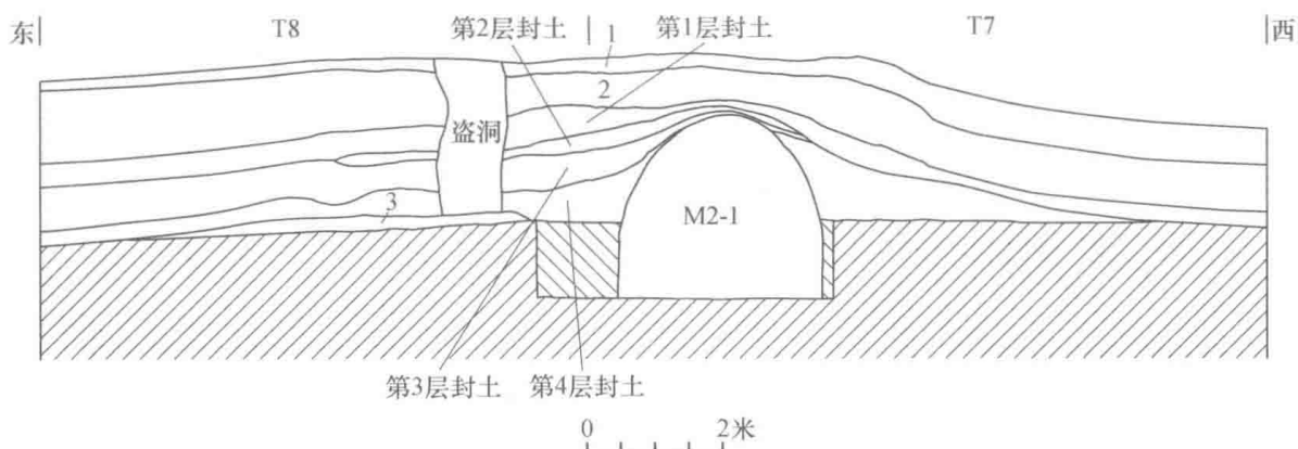
图二 T7、T8南壁剖面图
