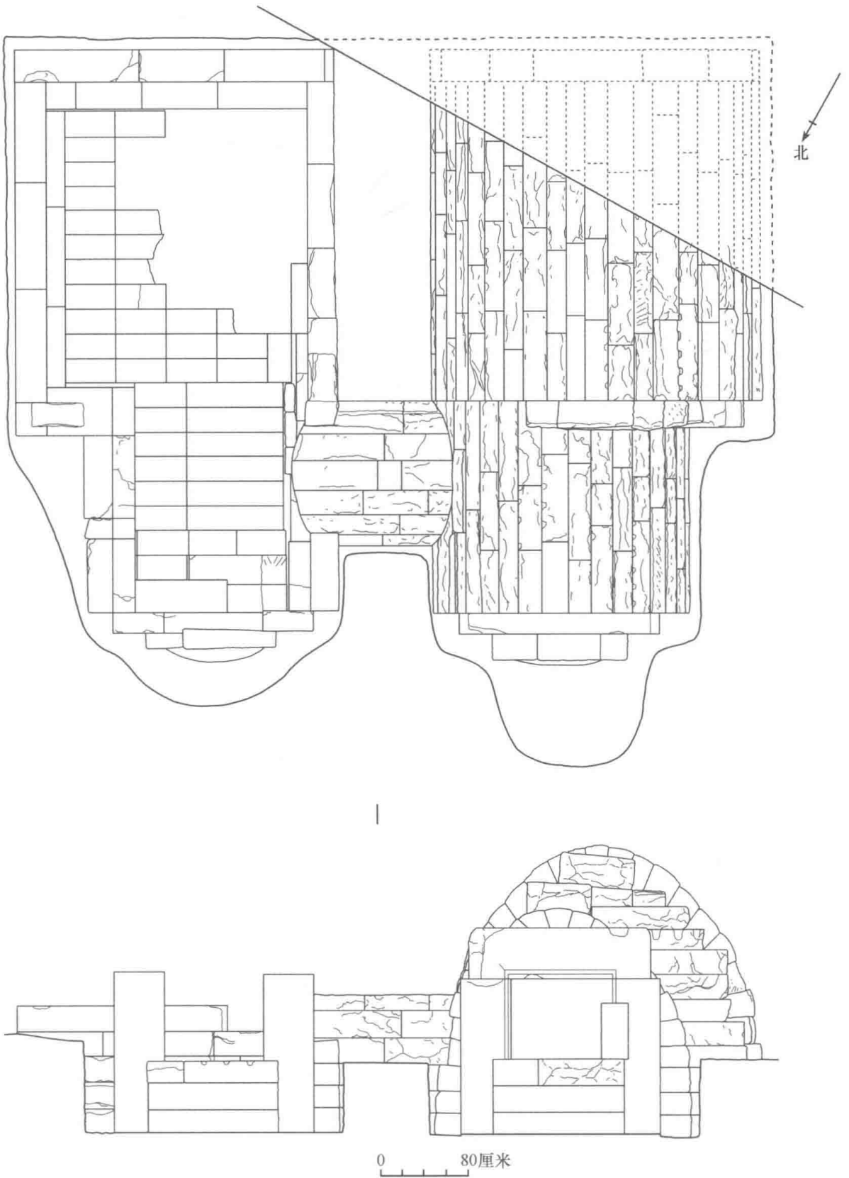
图三 M2正视、顶视图
