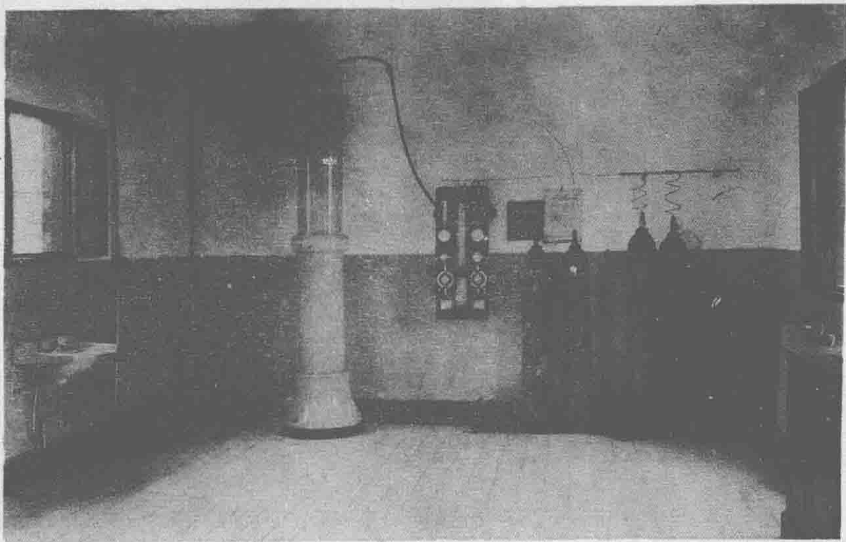
水廠加氯消毒設備
