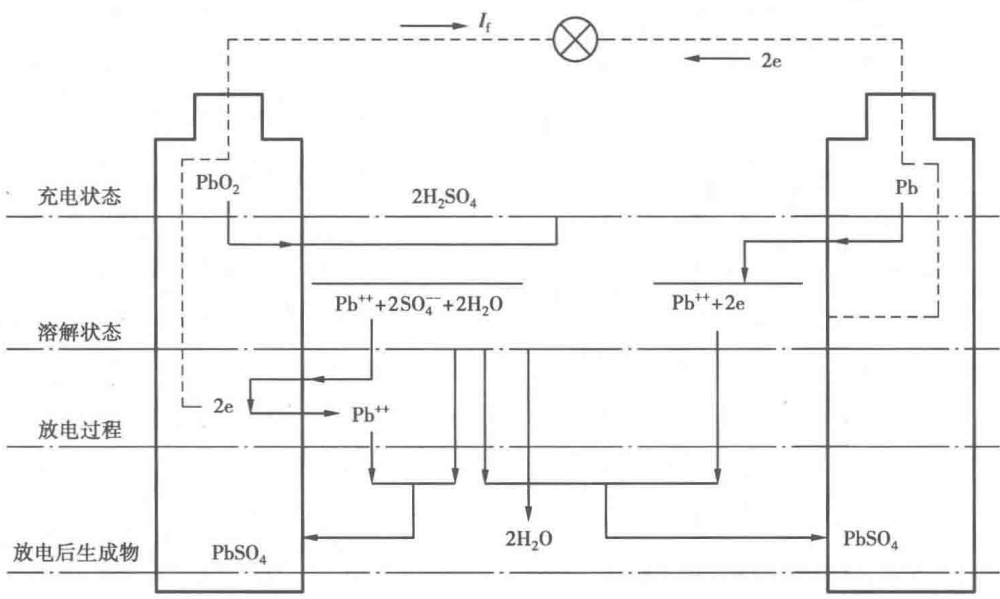
图 1-3 铅蓄电池放电过程
