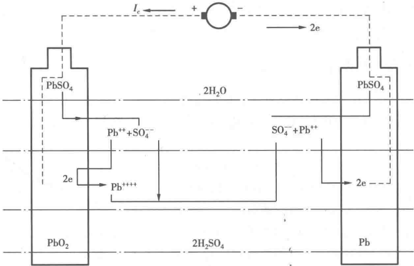
图 1-4 铅蓄电池的充电过程
