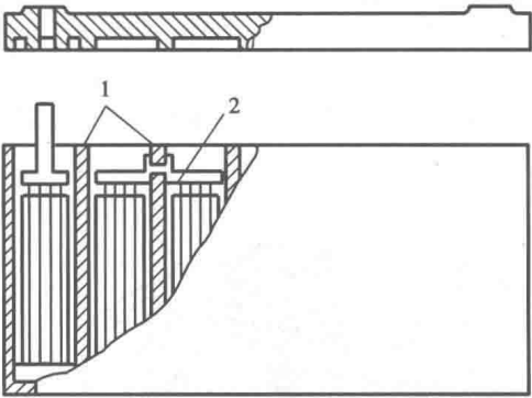
图 1-2 单格电池之间的穿壁焊示意图 1—间壁 2—联条
