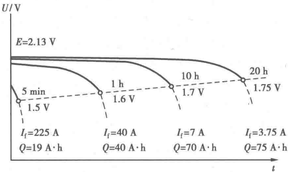
图 1-7 放电电流对容量的影响
