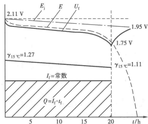
图 1-6 蓄电池放电特性
