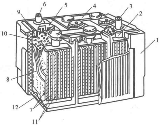
图 1-1 蓄电池的构造
