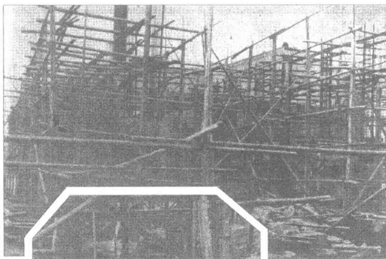
上 工作中之擴充廠房工程 中 擴充廠房工程中之 骨架雛形 下 擴充廠房工程中之 迴冷水塔之石基
