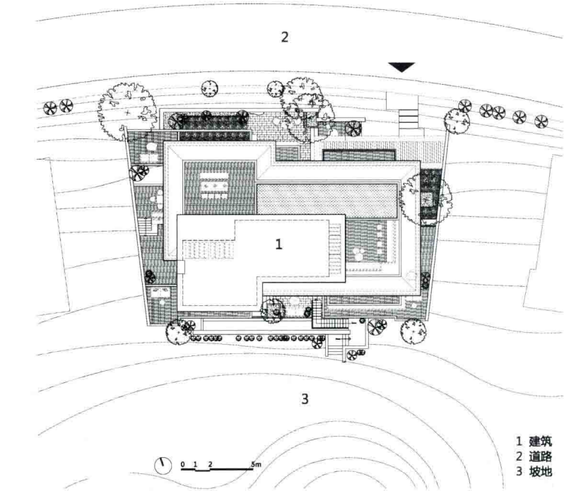
总平面图
