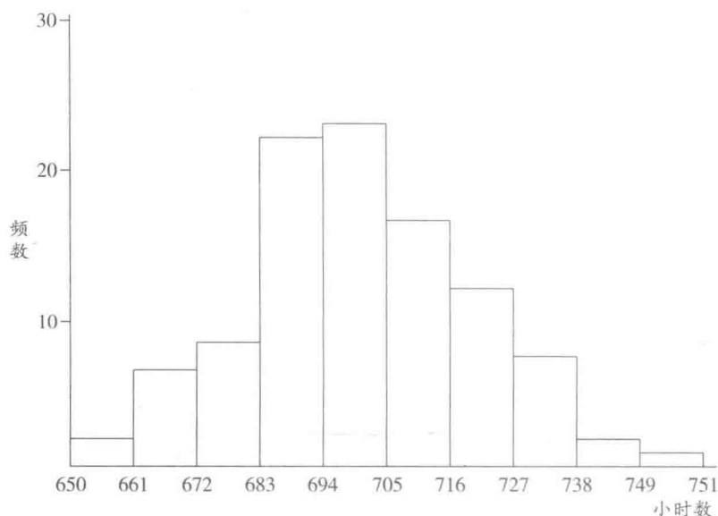
图 1-1 100只灯泡使用寿命频数分布图
