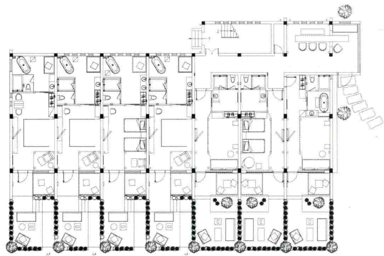
一层平面图
