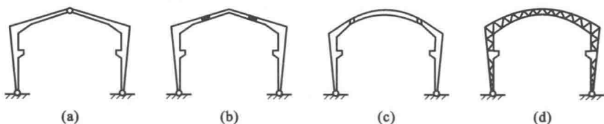
图 1.6 门式刚架
