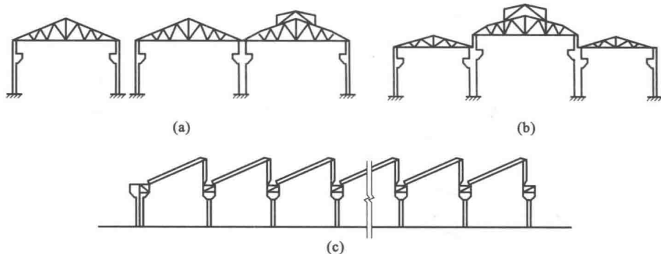
图 1.5 钢筋混凝土排架结构厂房
