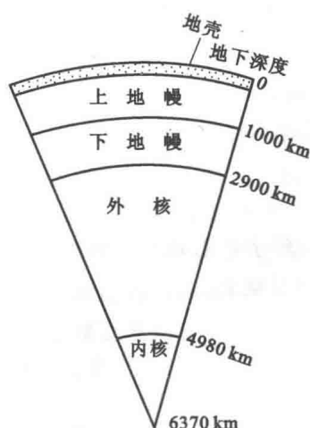
图 1.4 地球内部构造
