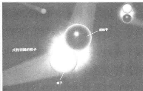
成对消灭的粒子——粒子、反粒子
