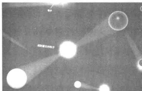
成对产生的粒子
