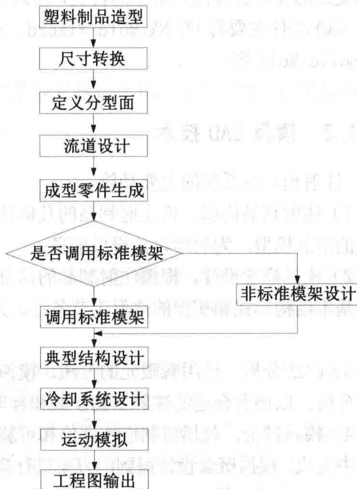
图 1-2 模具结构详细设计的流程图
