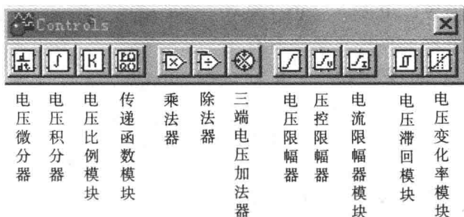
图 1-15 控制器件库
