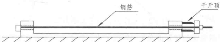
(1) 张拉钢筋
