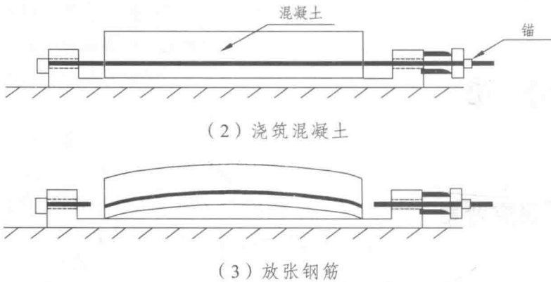
图 1.1 先张法主要施工工序
