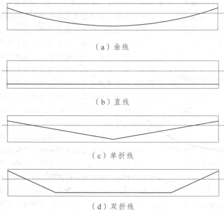
图 1.3 简支梁预应力钢束布置形式
