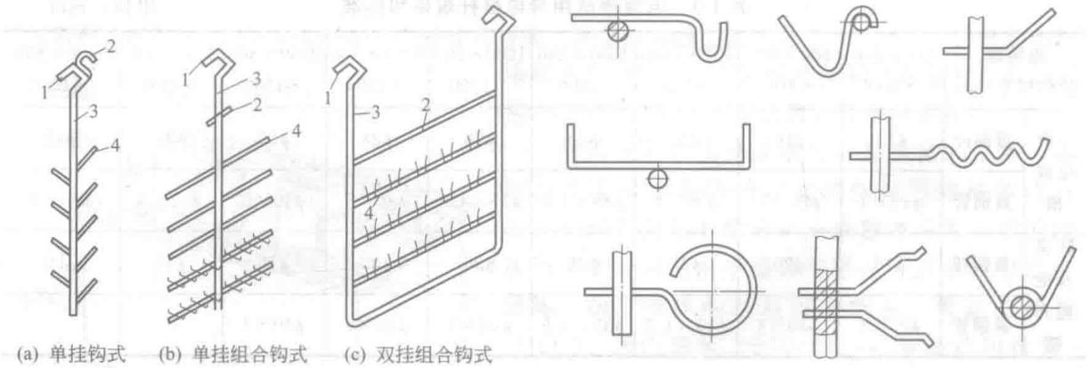
图 1-3 电镀挂具形式和结构
