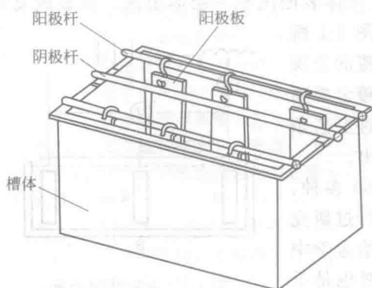
图 1-2 常规电镀槽结构
