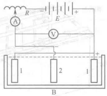
图 1-1 电镀装置示意
