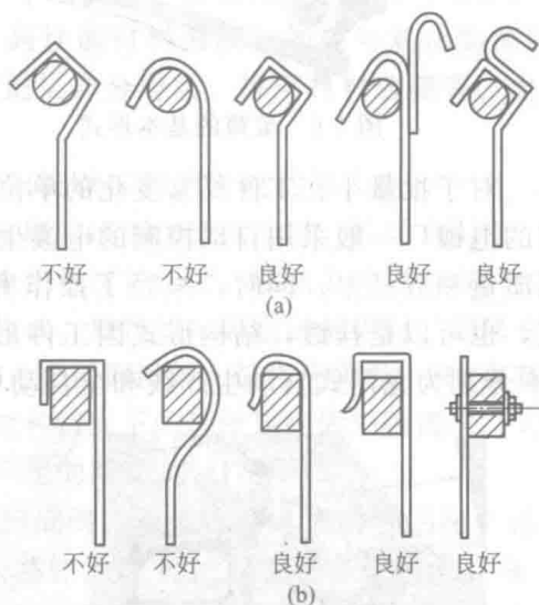
图 1-5 挂具悬挂方法的比较
