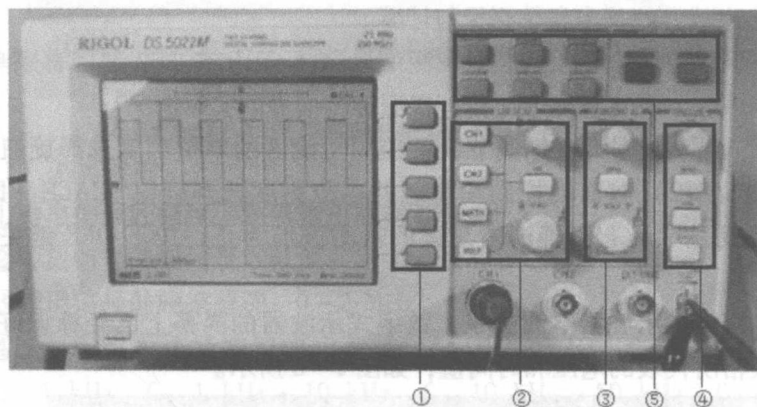
图 1-5 DS5022M 数字式示波器操作面板
