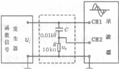
图 1-9 两波形间相位差测量电路
