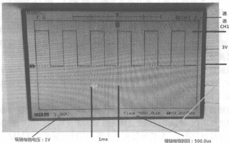
图 1-6 数字式示波器信号参数测量与计算
