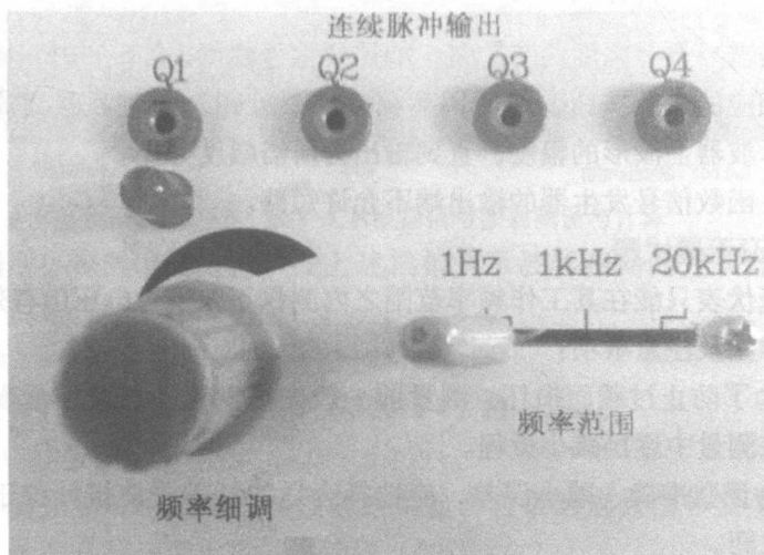
图 1-8 KHD-2 型数字电路实验台自带脉冲信号源
