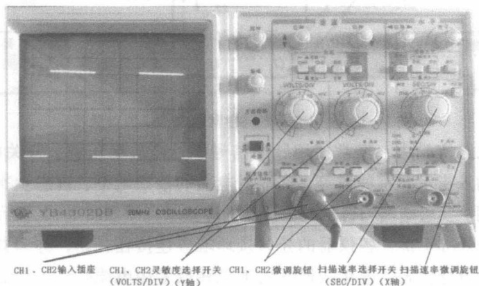
图 1-3 双踪示波器 YB4320 操作面板
