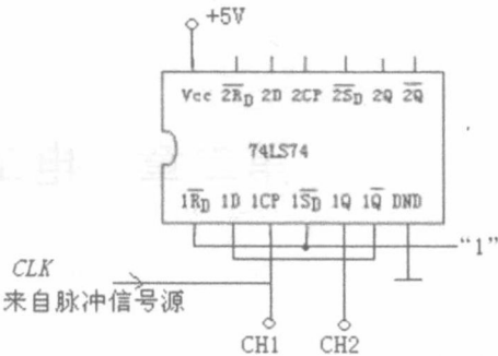
图 1-10 D→T' 电路连接图
