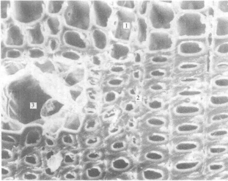
图 1-2 马尾松横切面(SEM × 300)
