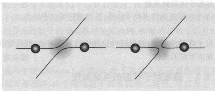
图 1.1 两个粒子的碰撞过程示意图 (阴影区表示两个粒子的波函数有严重重叠)
