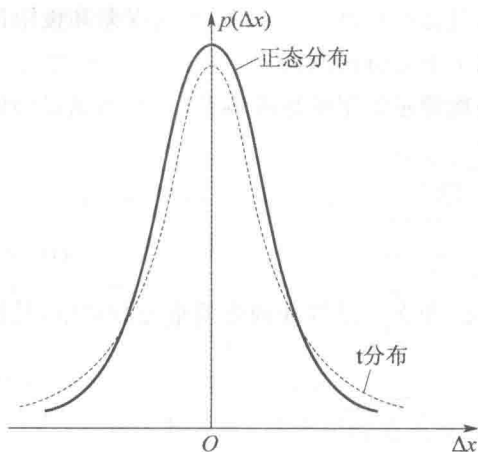
图 0-3 t 分布概率密度函数的曲线
