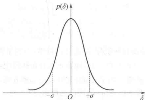
图 0-2 测量误差位于 (-\sigma \sim +\sigma) 范围的概率为 68.3%
