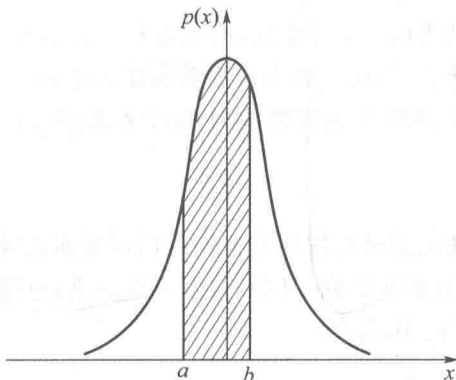
图 0-1 连续型随机变量的概率密度函数
