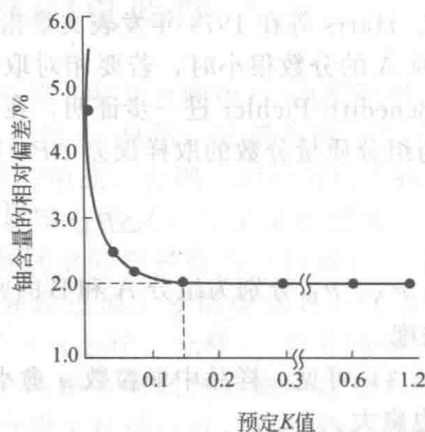
(b) 预定 K 值法选 K 值(原样480kg, d \leq 10\text{mm} )
