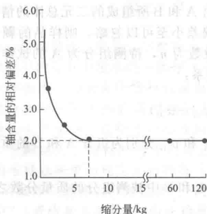
(a) 连续缩分法求 K 值
