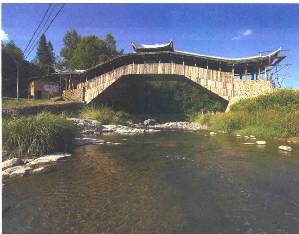
泰顺三座国保廊桥修复工程通过验收（图为工程开工现场、构件甄别归位、主体完工后的文兴桥）
