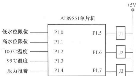
图 1-4 电加热锅炉单片机控制系统
