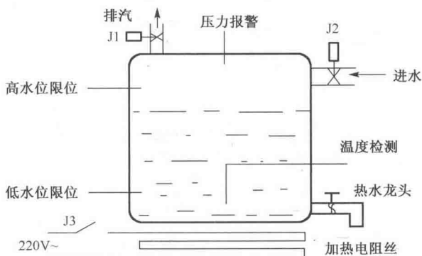
图 1-3 电加热锅炉
