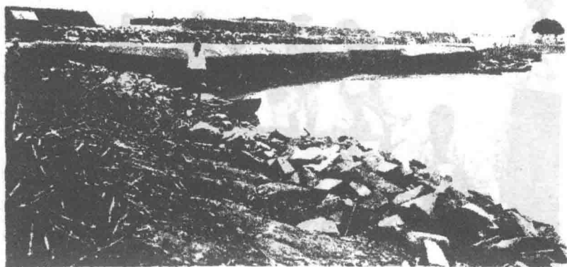
黃河朱口埽工
