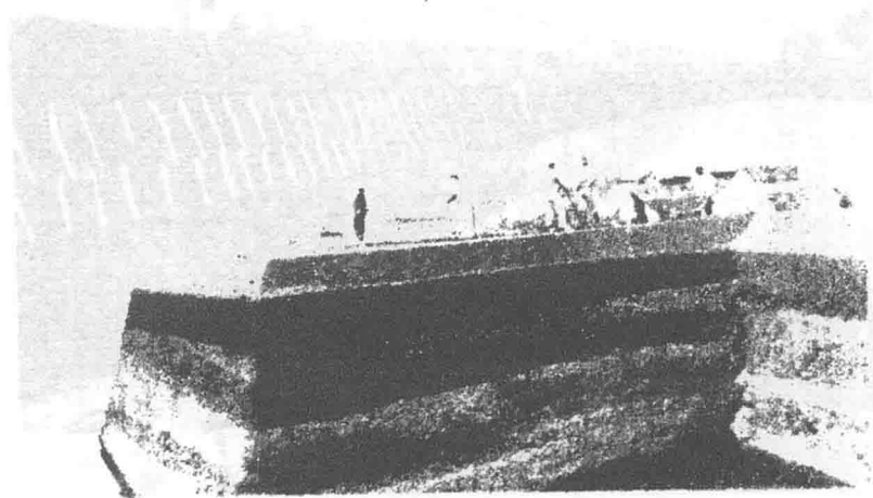
黃河劉莊埝工
