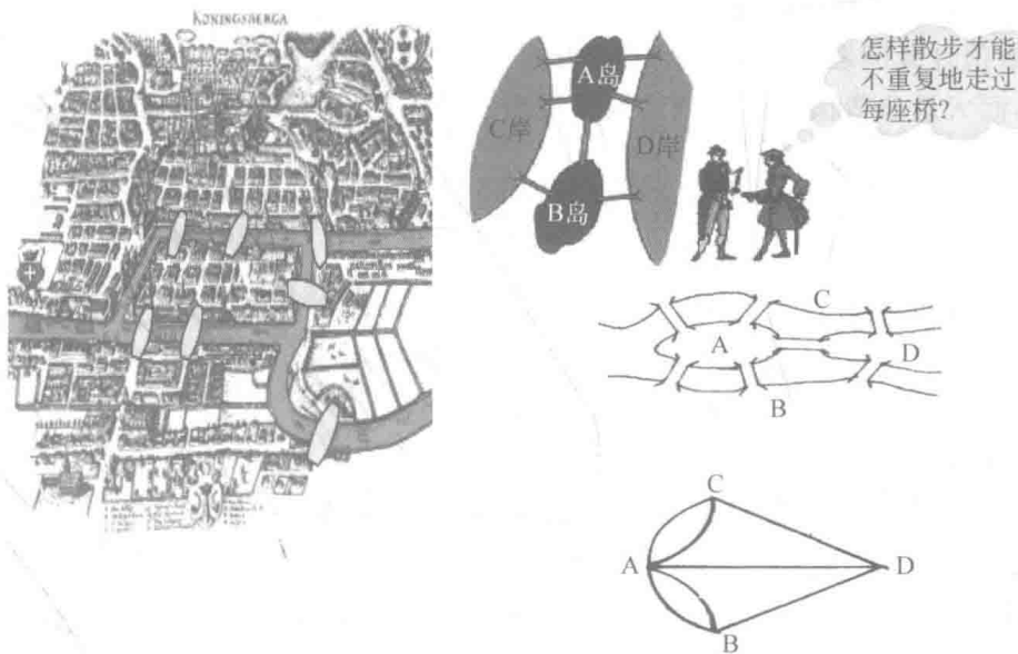
图 1.1 七桥问题图
