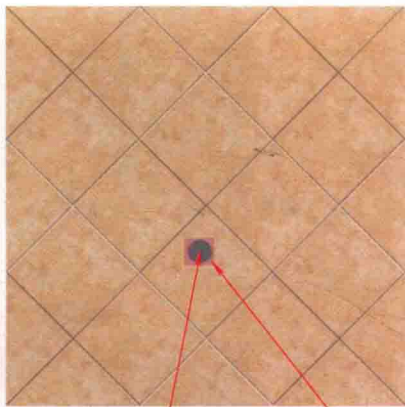
贴封植胶 第一次用6~8mm直径钻头预先打出小孔 然后用所需直径钻头进行扩孔 贴封箱胶
