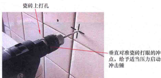
图 1-9 启动冲击锤打孔
