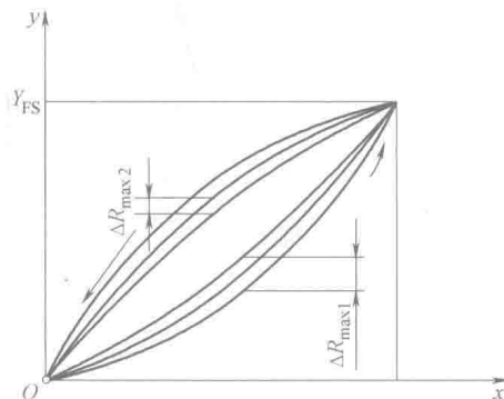
图 1.5 重复特性
