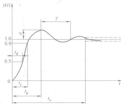
图 1.9 二阶传感器 ( \zeta < 1 ) 的时域动态特性
