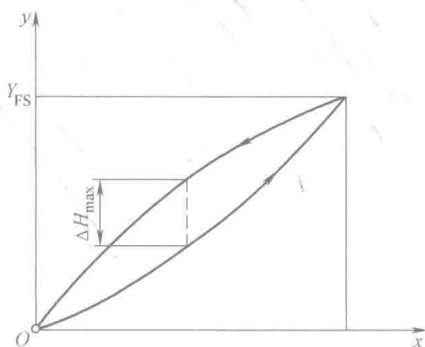
图 1.4 迟滞特性
