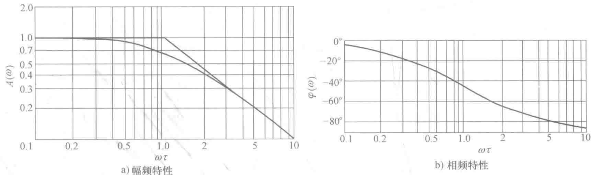
图 1.6 一阶传感器的频率响应特性曲线
