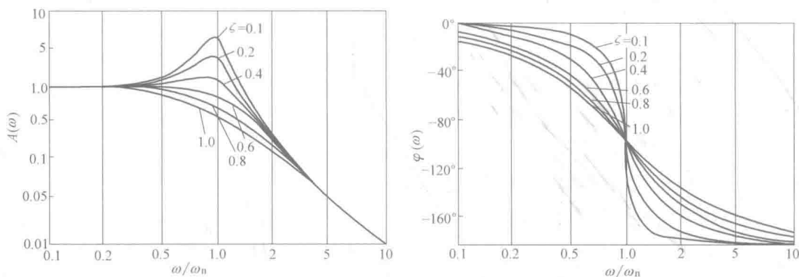
图 1.7 二阶传感器的频率响应特性曲线
