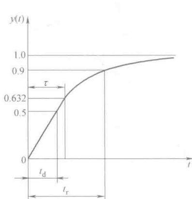
图 1.8 一阶传感器的时域动态特性
