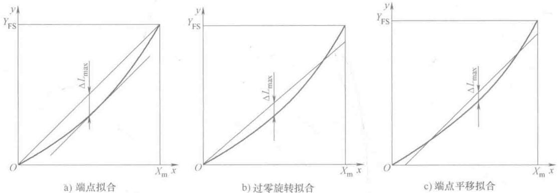
图 1.3 输入-输出特性线性化图
