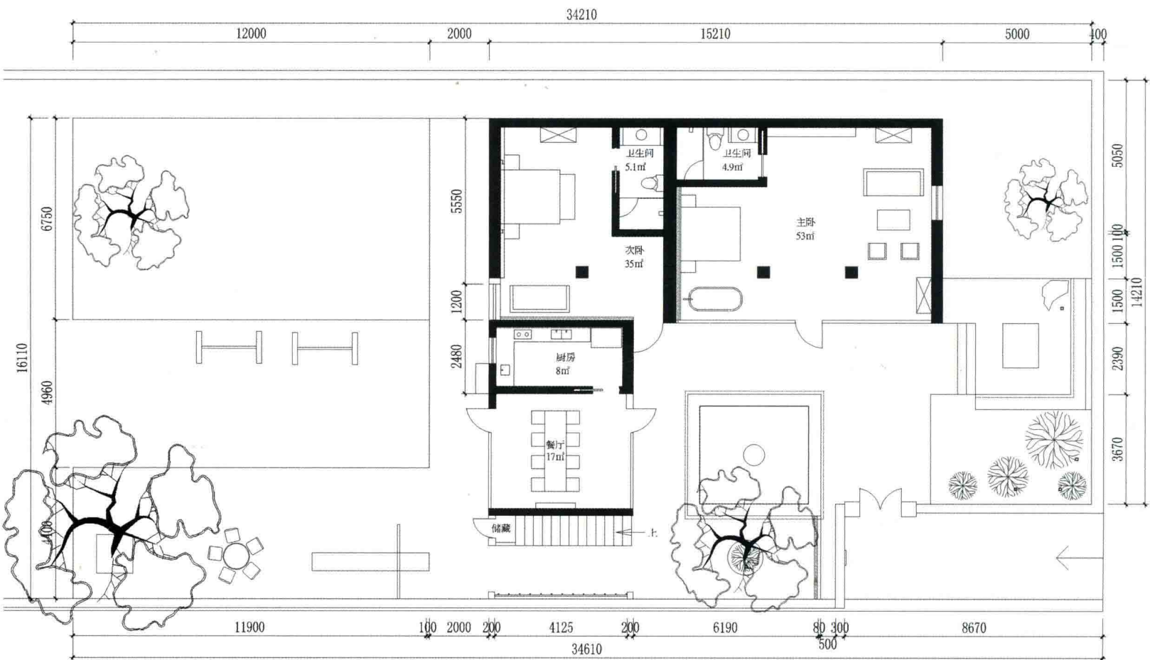
平面图
