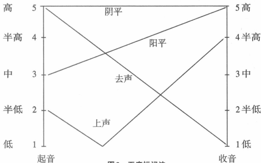
图2 五度标记法
