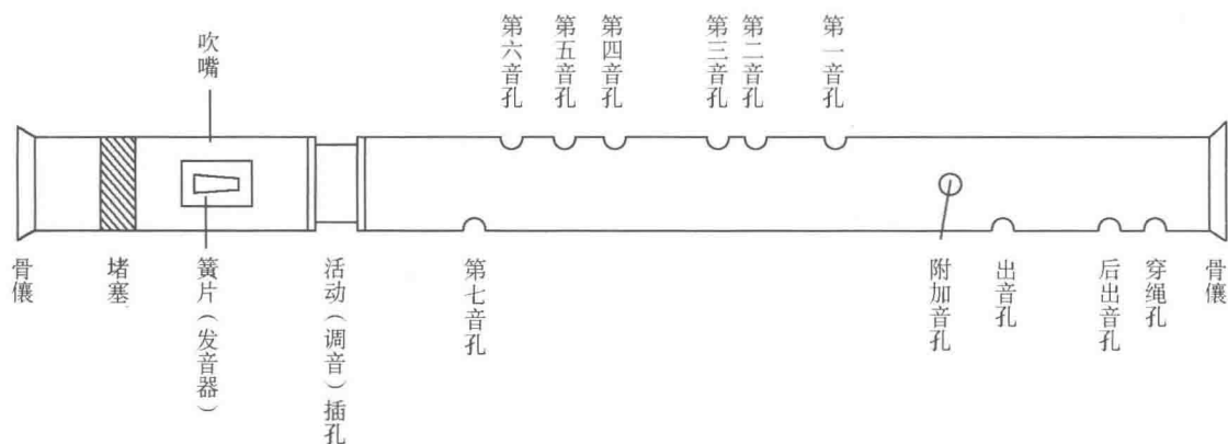
图 1-2 巴乌结构示意图
