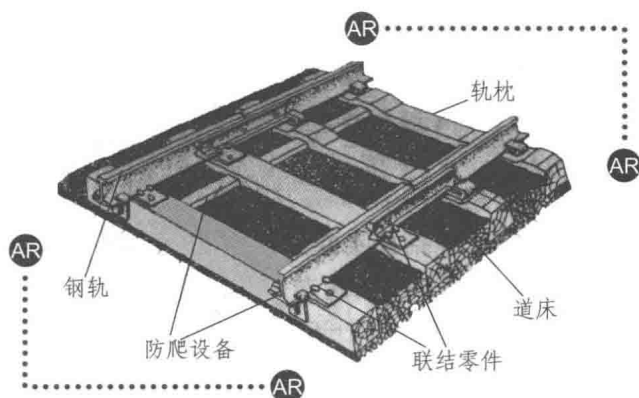
图 2.1 轨道的基本组成
