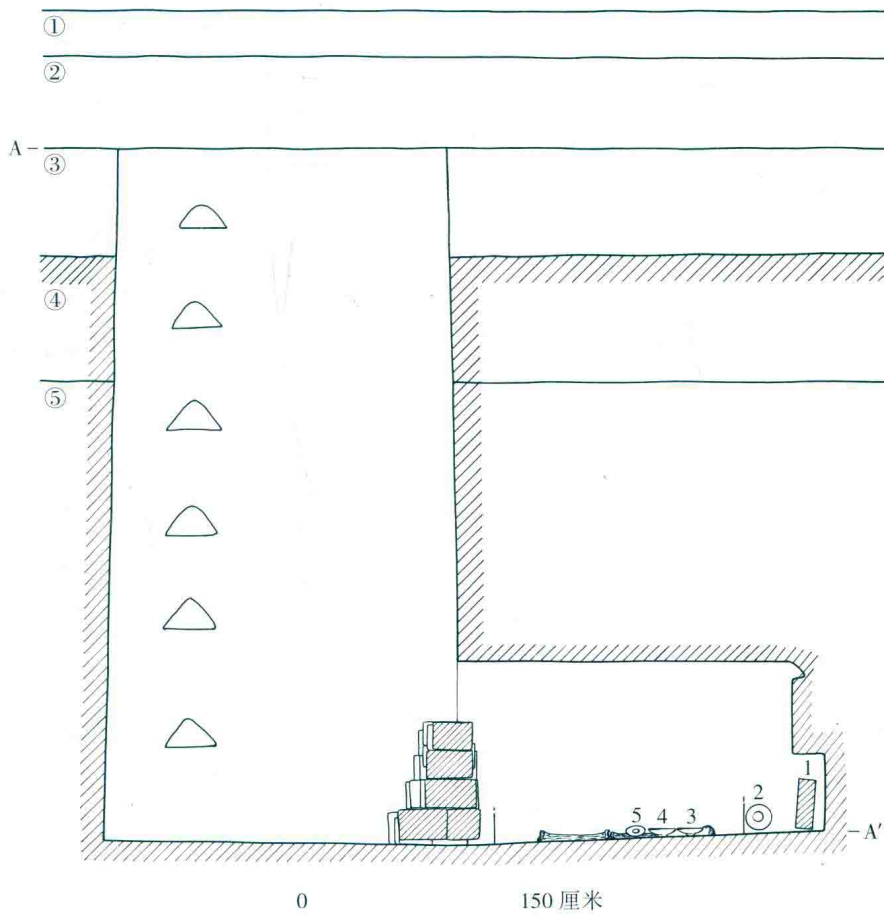
图 5-369 M16 纵剖面图
