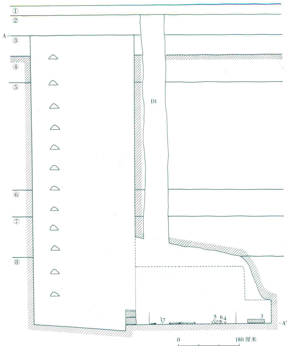
图 5-377 M17 纵剖面图
