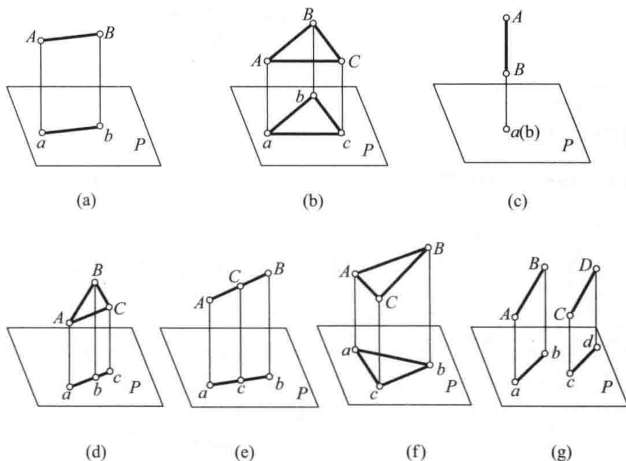
图 1-5 正投影的基本特性
