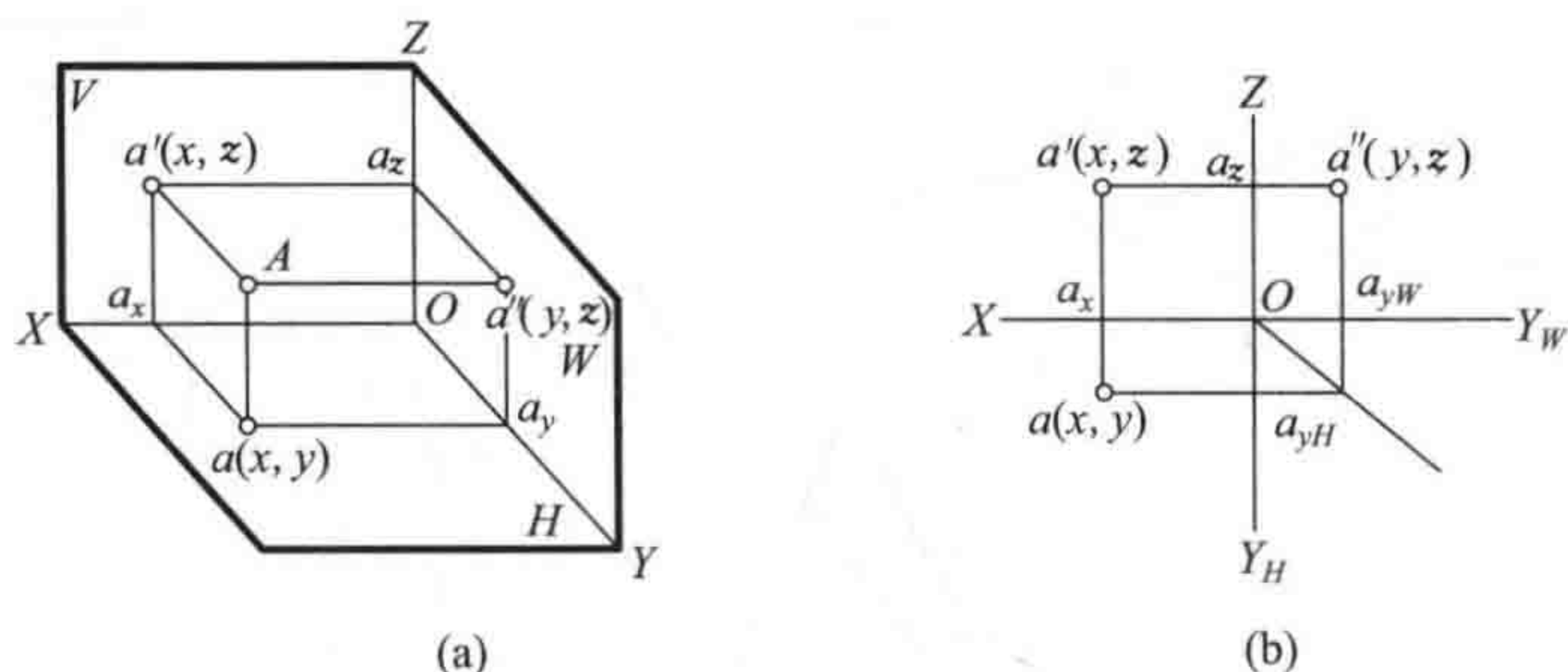
图 1-10 点的投影与坐标
