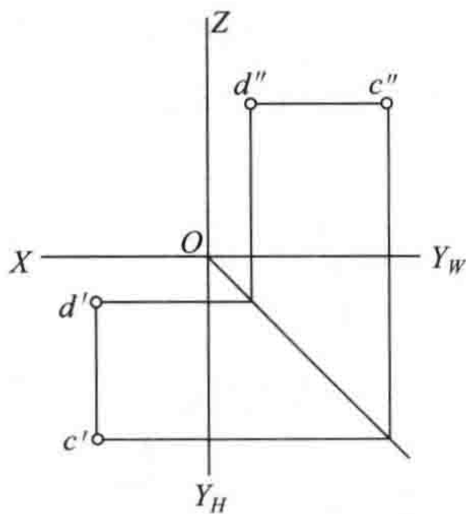
图 1-14 重影点的投影和可见性
