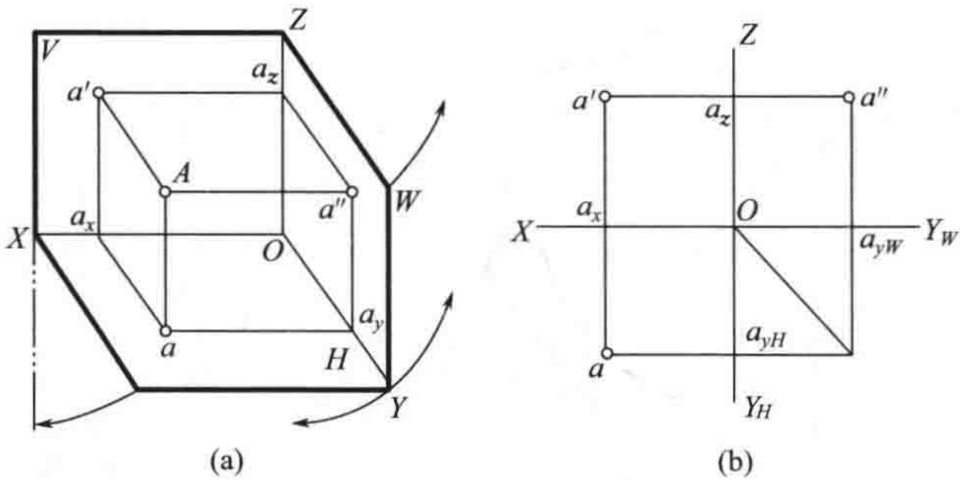
图 1-6 点的三面投影 (a) 空间状况；(b) 投影图
