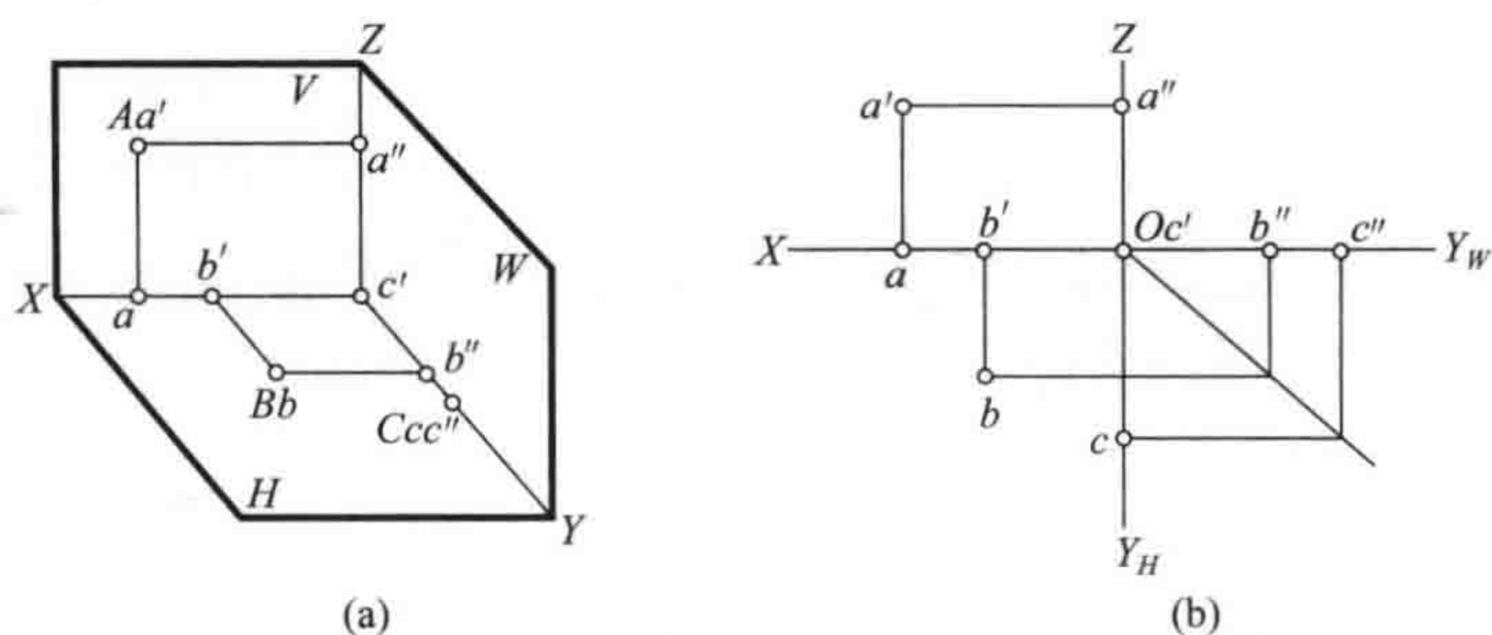
图 1-9 投影面、投影轴上的点的投影
