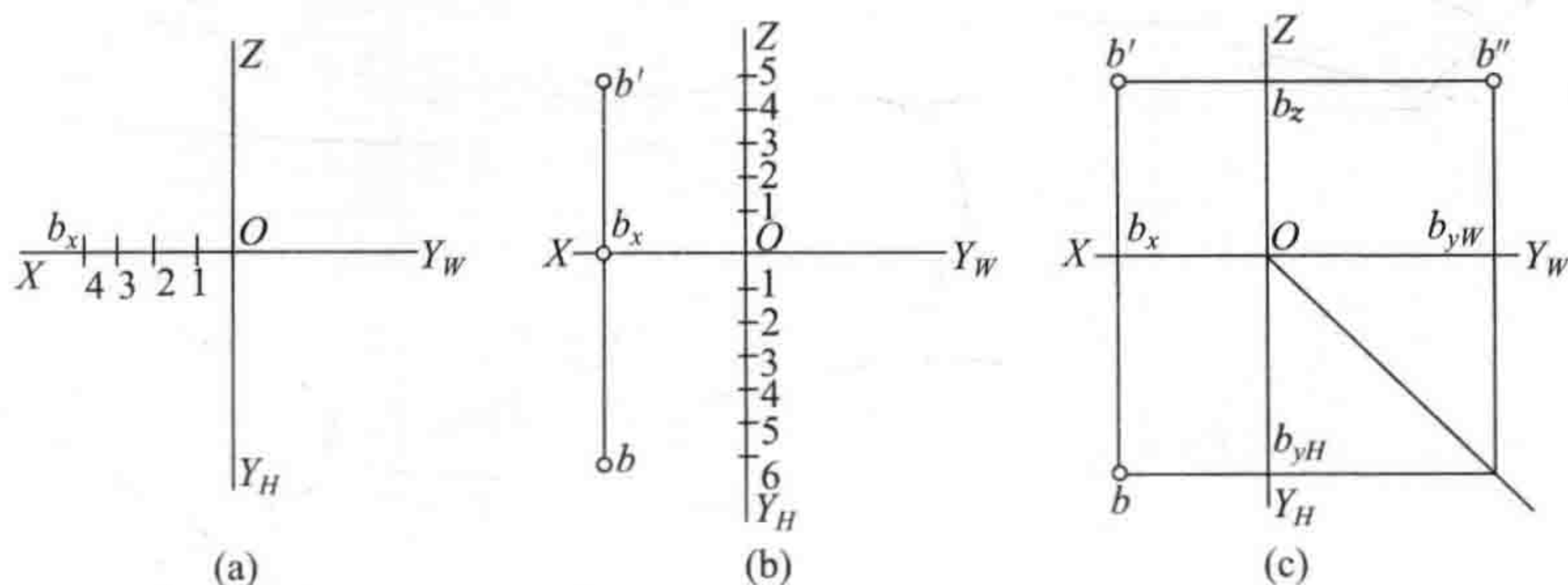
图 1-11 已知点的坐标，求点的三面投影
