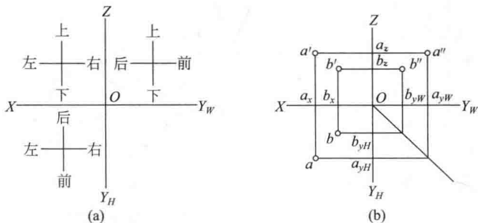
图 1-12 两点的相对位置
