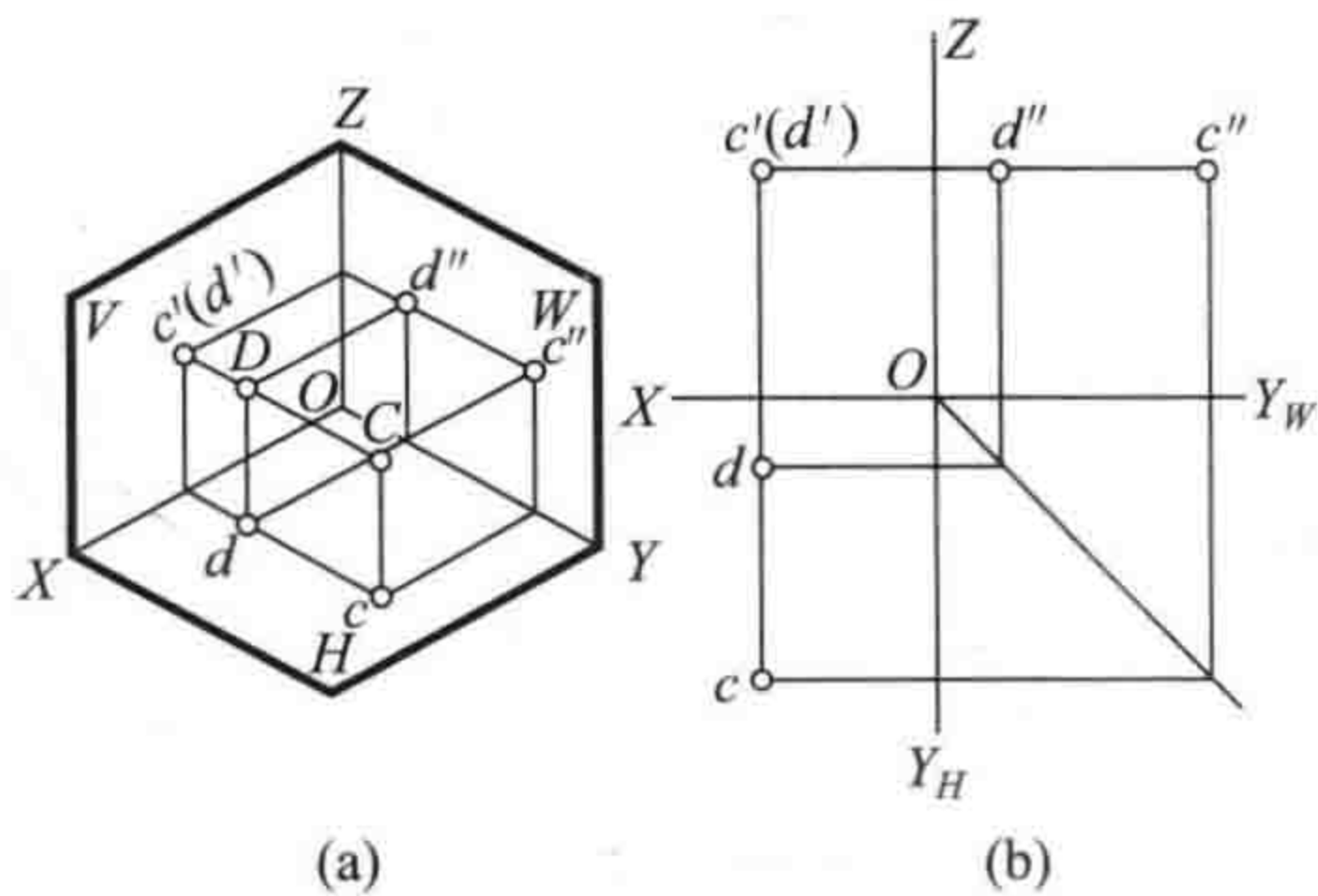
图 1-15 作图结果 (a) 重影点；(b) 作图结果
