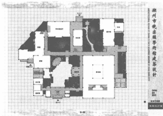
图7 饶宗颐学术馆首层平面图
