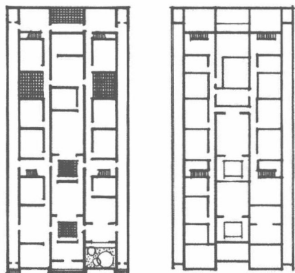
图2 西关大屋平面图
