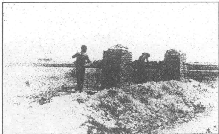
農夫取水方法之二——轆轤
