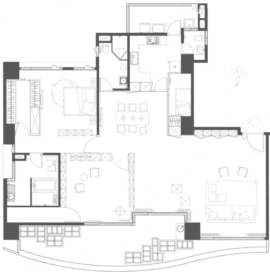
一层平面图
