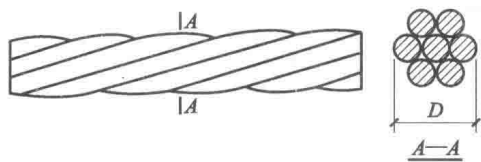
图 2-2 钢绞线的表面及截面形状
