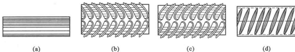
图 2-1 钢筋的表面形状
