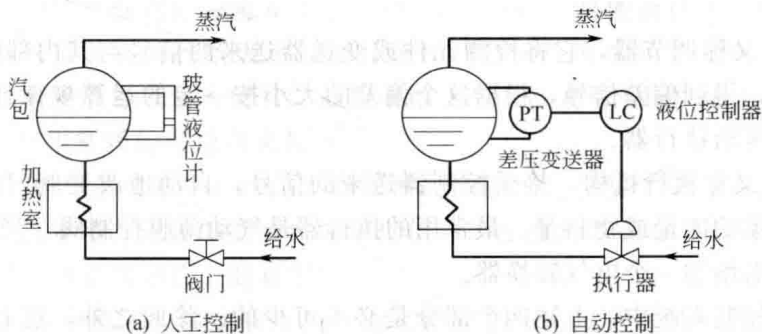
图 1-1 锅炉汽包水位控制示意图
