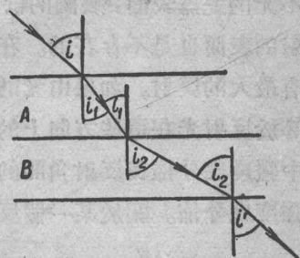
圖 4 通過二平面平行透明板時，光線的折射。
