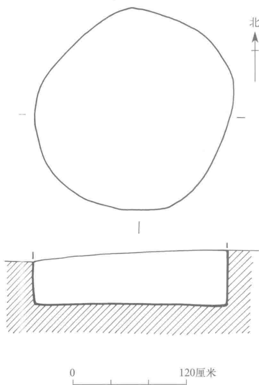
图6-14 04H32平、剖面图
