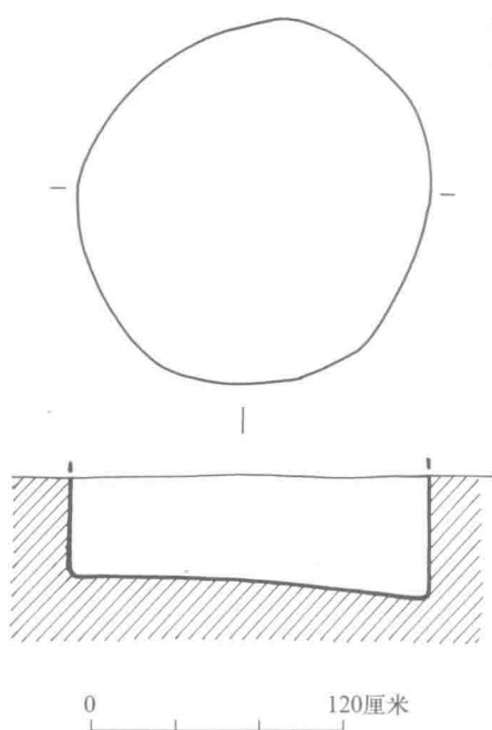
图6-12 04H14平、剖面图
