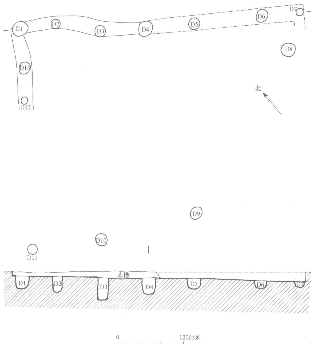
图6-8 04F3柱洞平、剖面图
