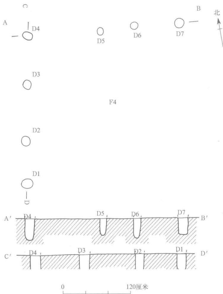
图6-9 04F4柱洞平、剖面图
