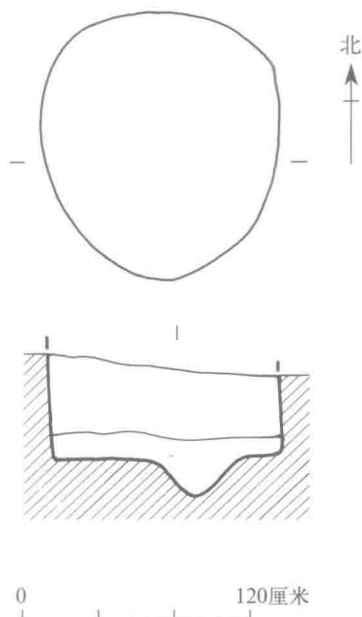
图6-13 04H23平、剖面图
