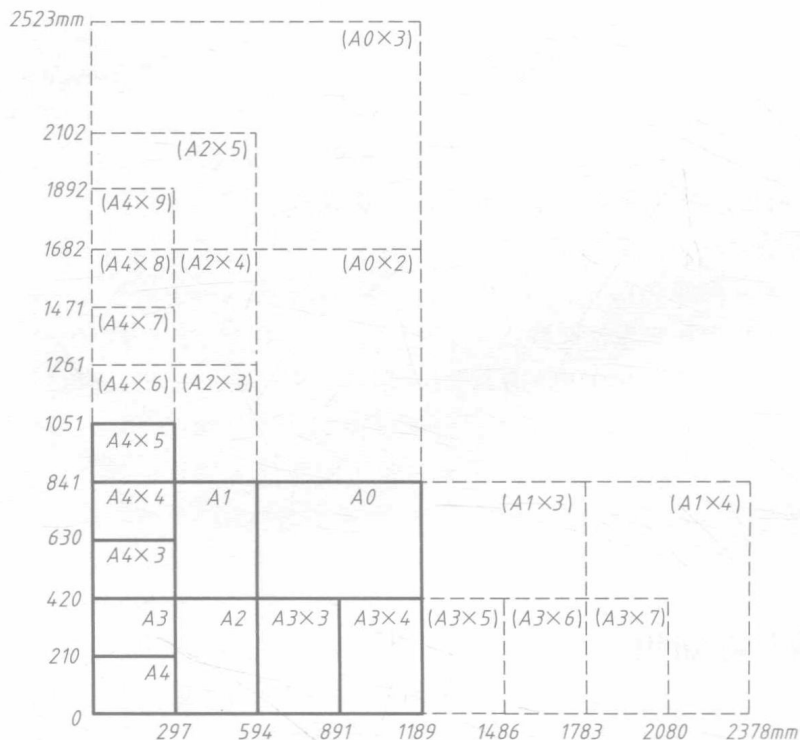
图 1-1 图纸幅面的尺寸
