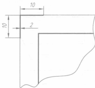
b) 剪切符号二
