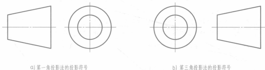
图 1-9 投影符号的画法
