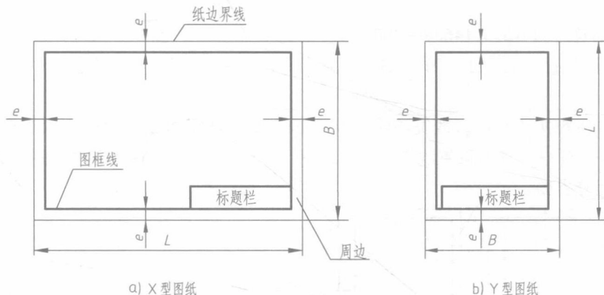
图 1-3 无装订需求的图框格式
