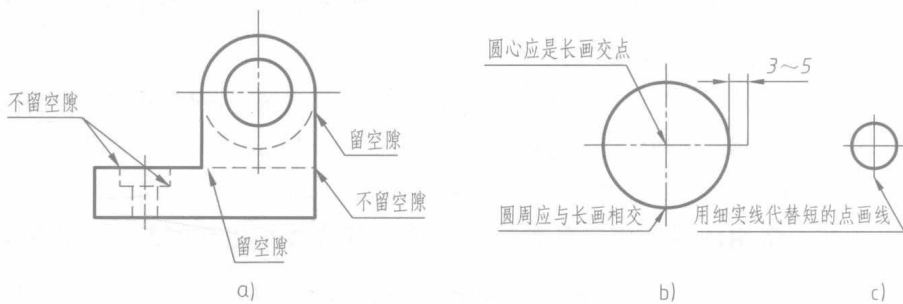
图 1-13 虚线连接处画法
