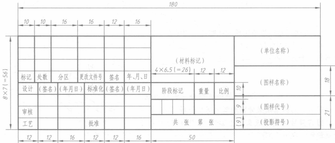
图 1-4 标题栏格式和尺寸
