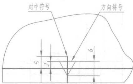
图 1-7 对中符号与方向符号
