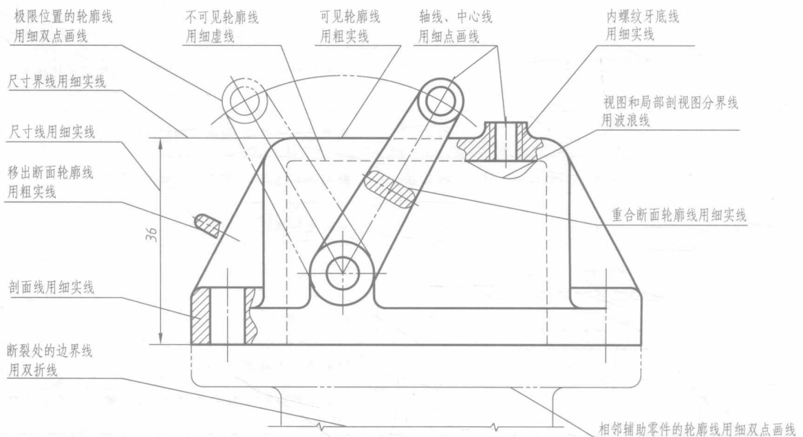
图 1-14 各种线型在图样中的运用
