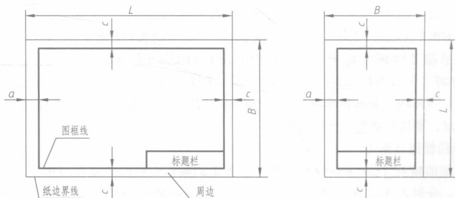
a) X型图纸
