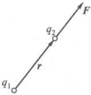
图 10-1 点电荷 q_2 所受库仑力 (设 q_1 与 q_2 同号)
